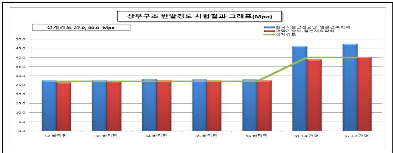
【그림 18.4.2】 상주방향 상부구조 반발경도시험 측정결과
