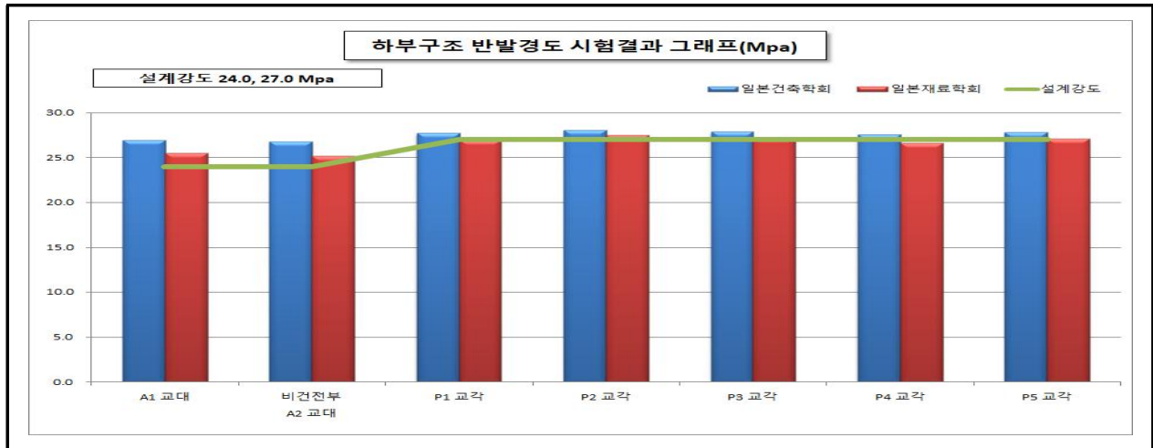
【그림 18.4.5】 영천방향 하부구조 반발경도시험 측정결과
