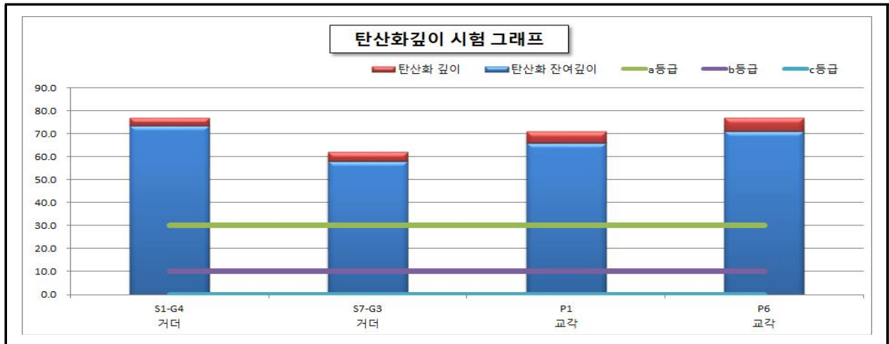
【그림 18.4.7】 영천방향 탄산화 깊이 측정결과
